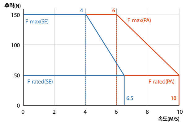
모터 추력 및 속도특성(Thrust & velocity of motor)
