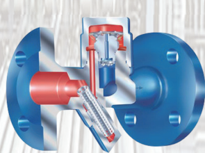
디스크 스팀 트랩
