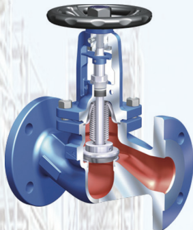
벨로우즈씰 스톱밸브
