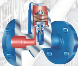
바이메탈 스팀 트랩
