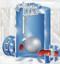
응축수 회수펌프
