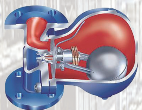
볼플로트 스팀 트랩
