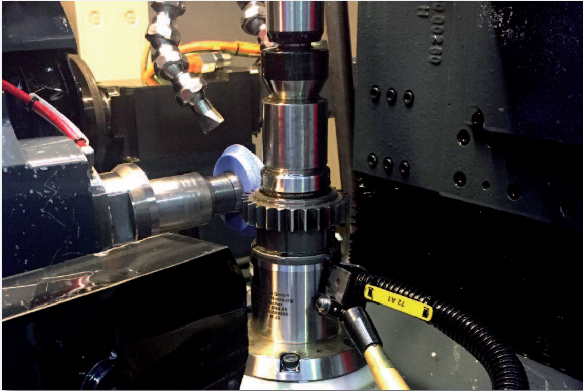
치가공
