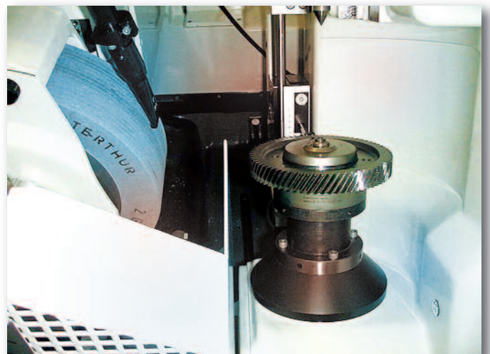
... 연마 공정용
