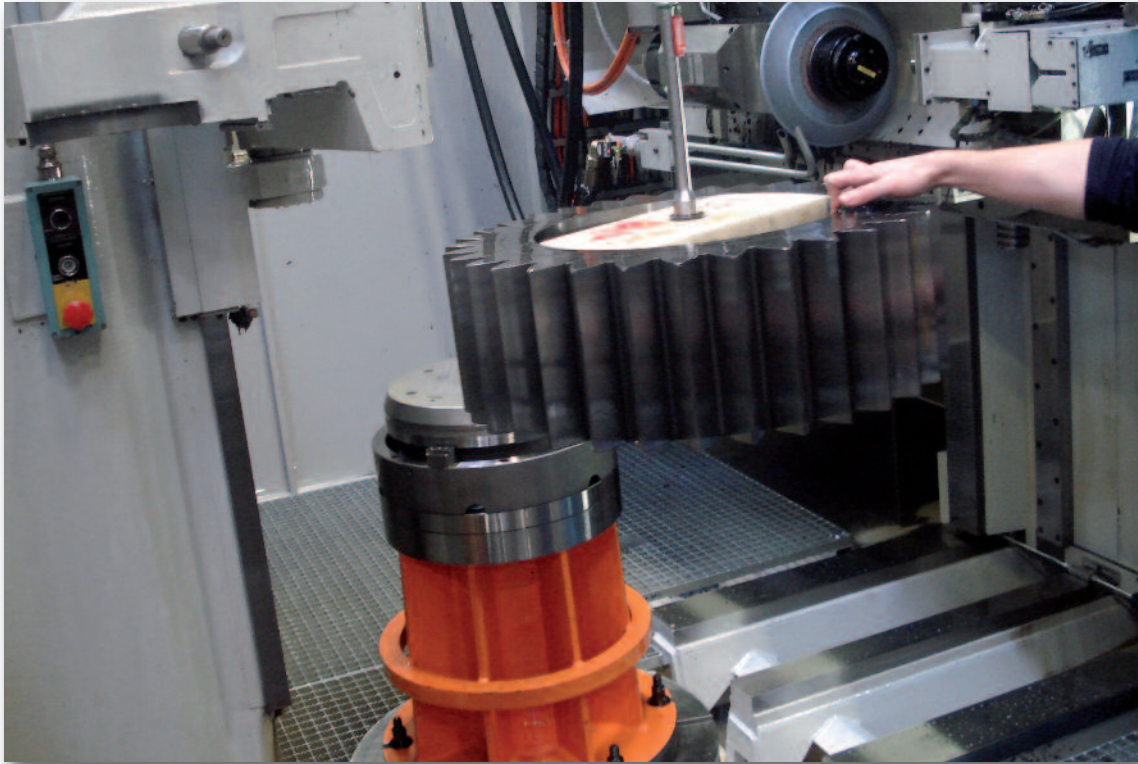
연마
