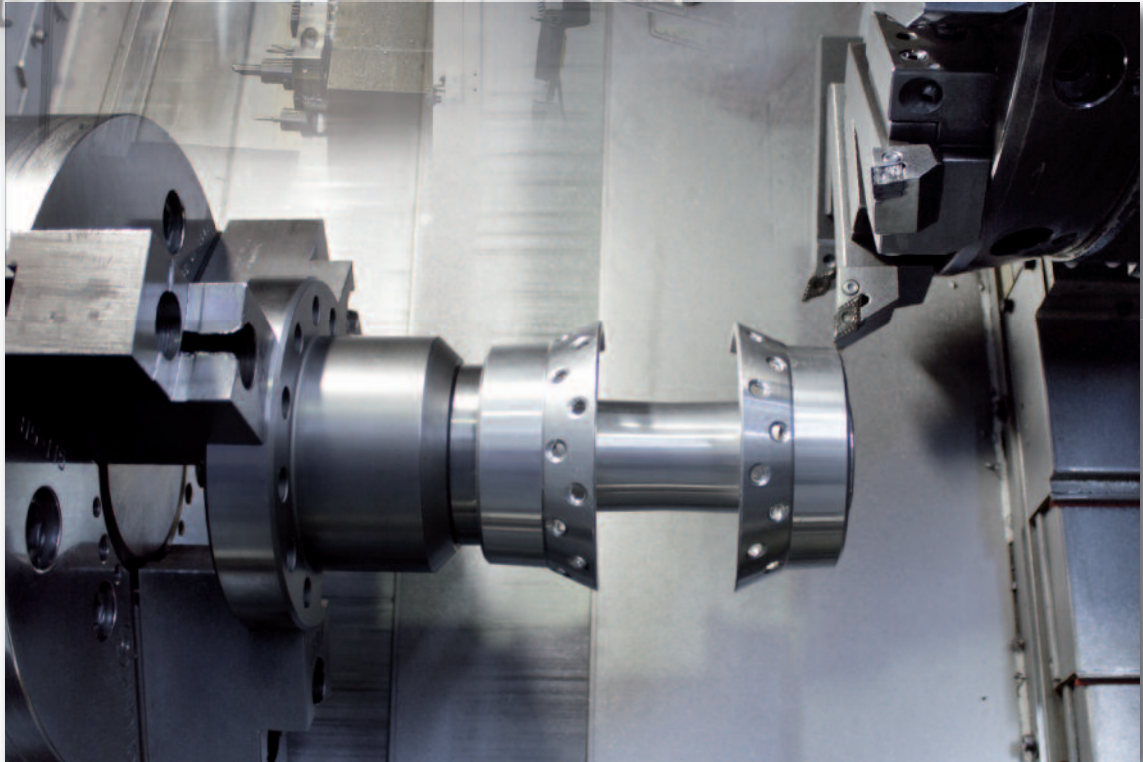
선반
