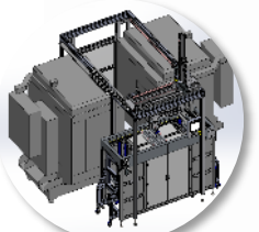
굴삭기 유압 동력배분 샤프트 밀링/선반라인 장비 설계
