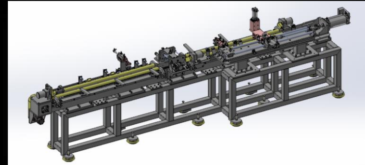
<PIPE INSERT MACHINE>
