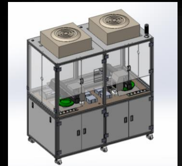
<BARREL ALIGN MACHINE>
