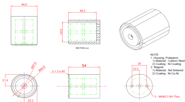
<Dimension : SFMV-L54-S10-F20>
