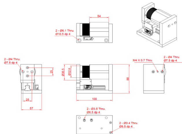
<Dimension : SFSV-L54-S10-F20>
