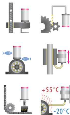
그리스 타입과 오일타입의 Simalube 자동주입기
